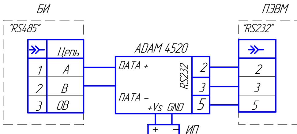
Рисунок 2.3 Схема электрическая соединений БИ анализатора АНКAT 7655-03 с ПЭВМ
