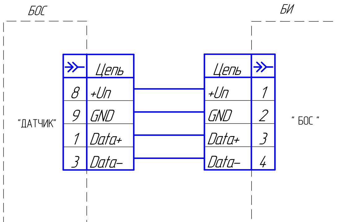
Рисунок 2.1 - Схема электрическая соединений БОС с БИ анализатора АНКAT 7655-02
